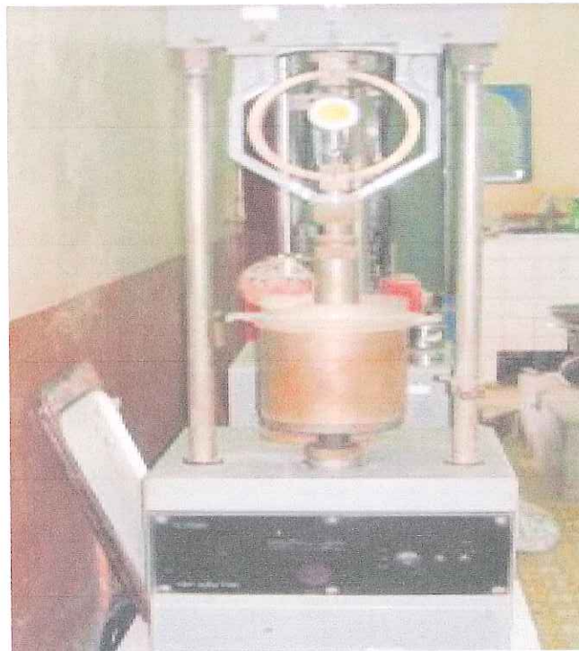
THIẾT BỊ NÉN CBR
